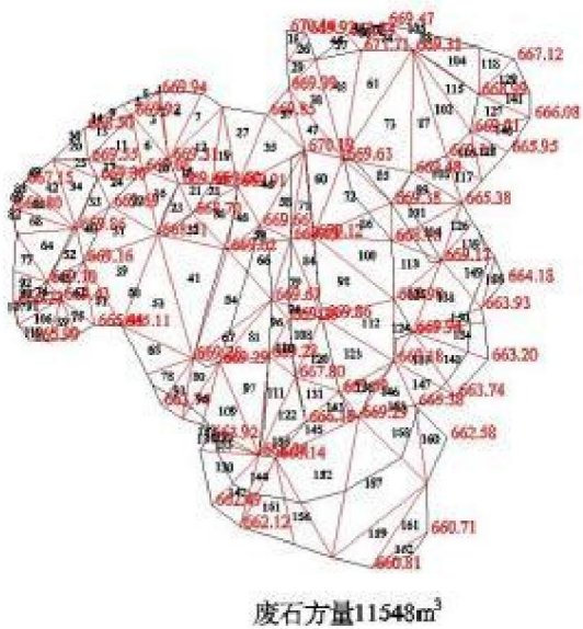
图4-2 SJ1废石堆放场方量三角网法计算成果图
